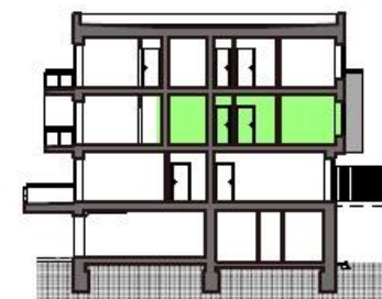
ŘEZ OBJEKTEM C2
