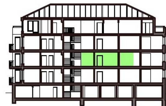
ŘEZ OBJEKTEM A-A
