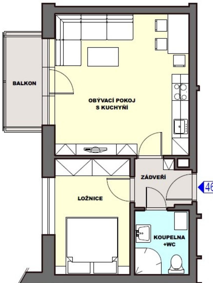
SCHEMA OBJEKTU
