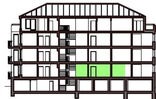
ŘEZ OBJEKTEM A-A
