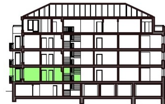
ŘEZ OBJEKTEM A-A
