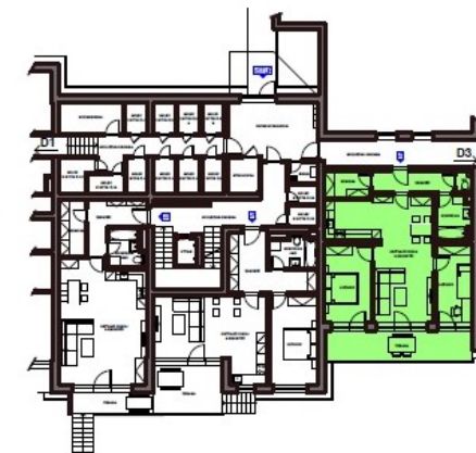
SCHEMA OBJEKTU
